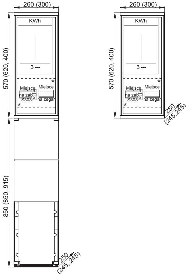
Przykład montażu szafy pomiarowej do słupa
